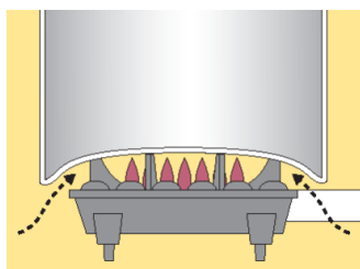
【二次空気不足の現象の例】
