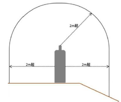
バルク貯槽
